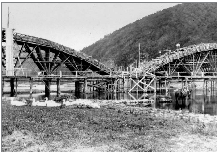
Betonování mostních oblouků, červenec až srpen 1928
